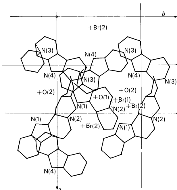
Fig. 9. Vue partielle de l'empilement moléculaire.
