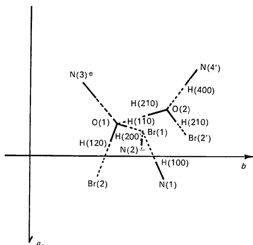
Fig. 8. Vue partielle des liaisons intermoléculaires.
